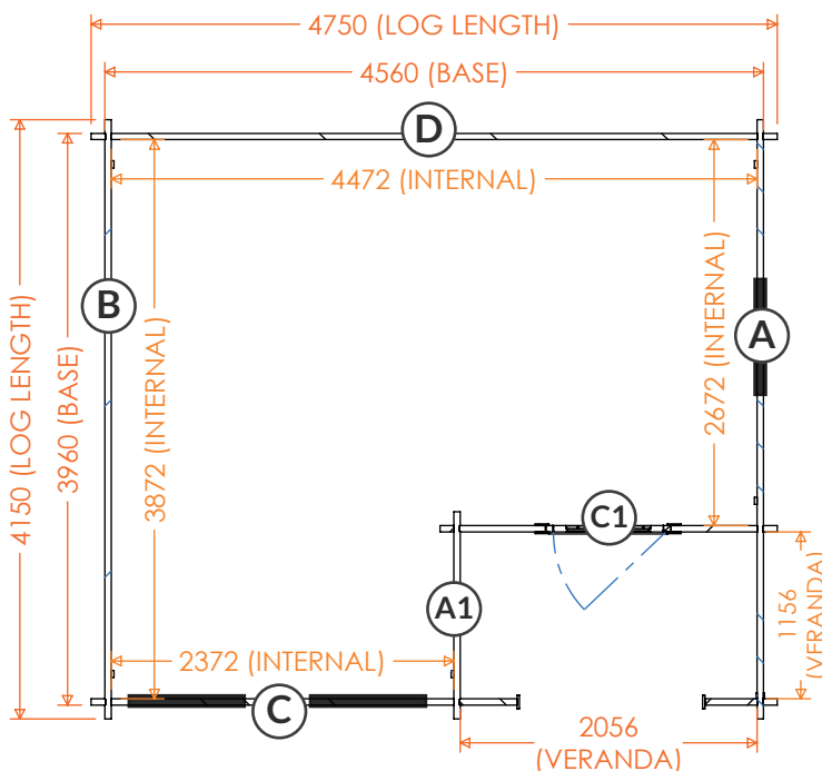
16x14w Amur 44mm 1614SIG-44
